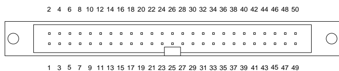
50 PIN 牛角接頭
