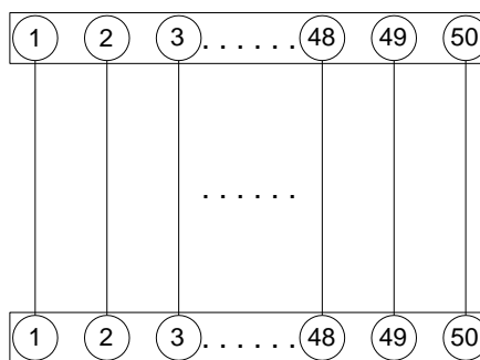
SCSI 50PIN 接頭
