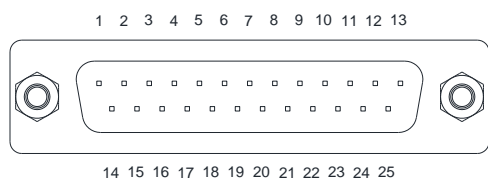
25 PIN D-SUB 接頭
