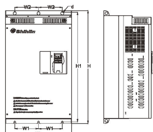
框架 G/H
